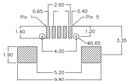
P.C.Board Layout
